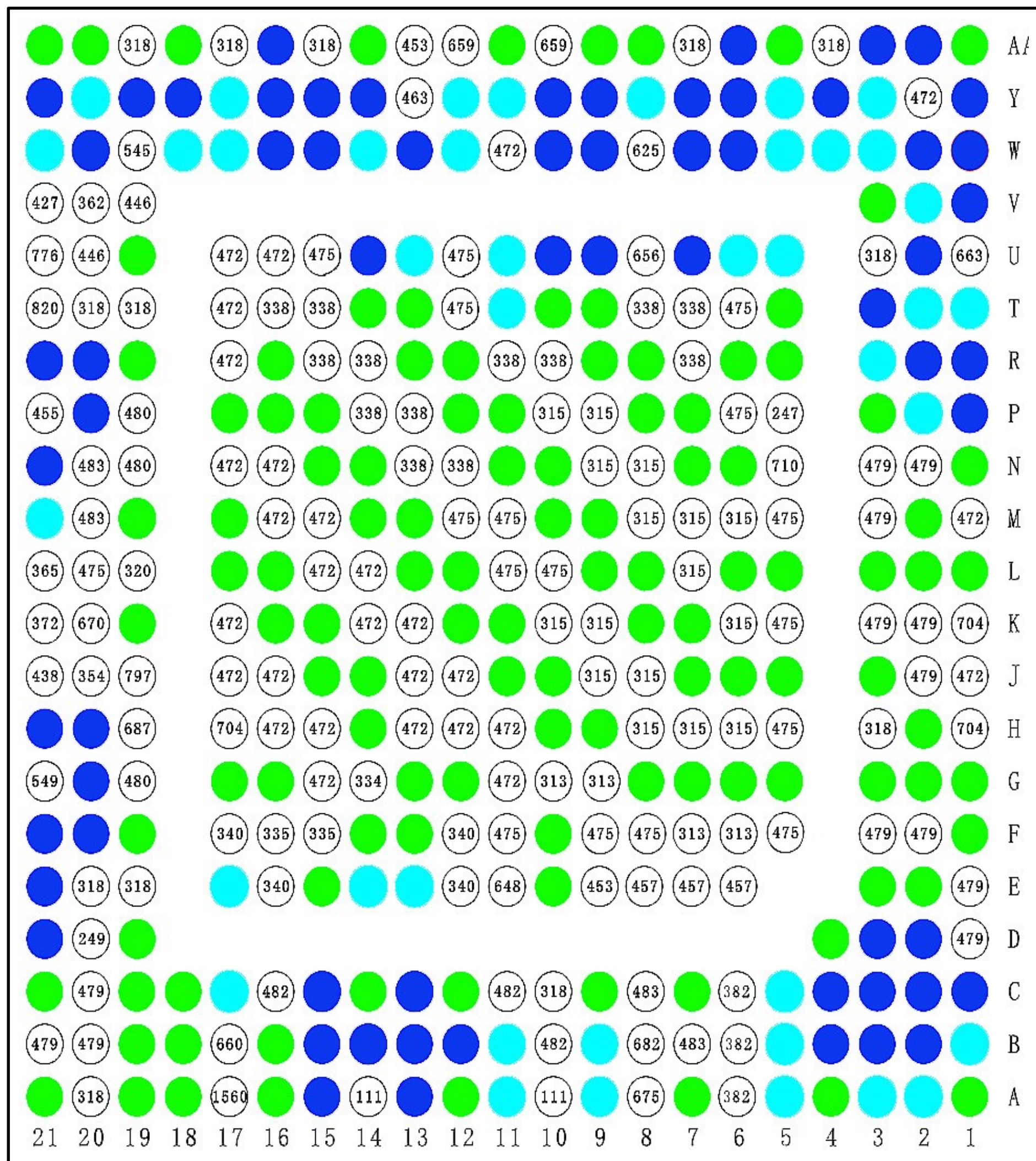
iPhoneX 基带CPU对地阻值图
